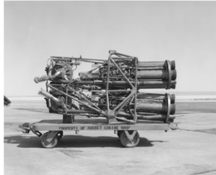
XLR-11 Engines.jpg
