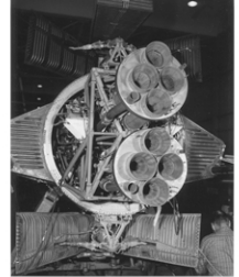
XLR-11 Installed.jpg
