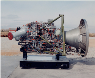
XLR-99 Engine_2.jpg
