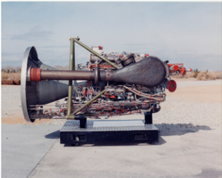
XLR-99 Engine_1.jpg
