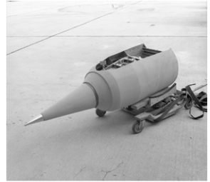
Ramjet On Cart 1.jpg
