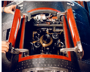
084. Startracker.jpg
