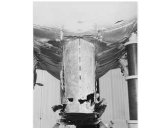
198. A-2 Damage.jpg
